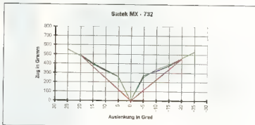
Für einen Joystick mit etwa 550 g maximalem Zug guter Verlauf (x).
